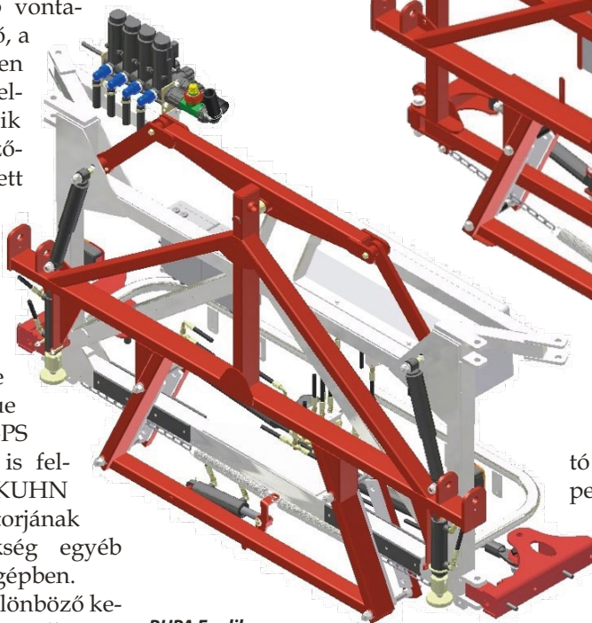
RHPA Equilibra keretfelfüggesztés
